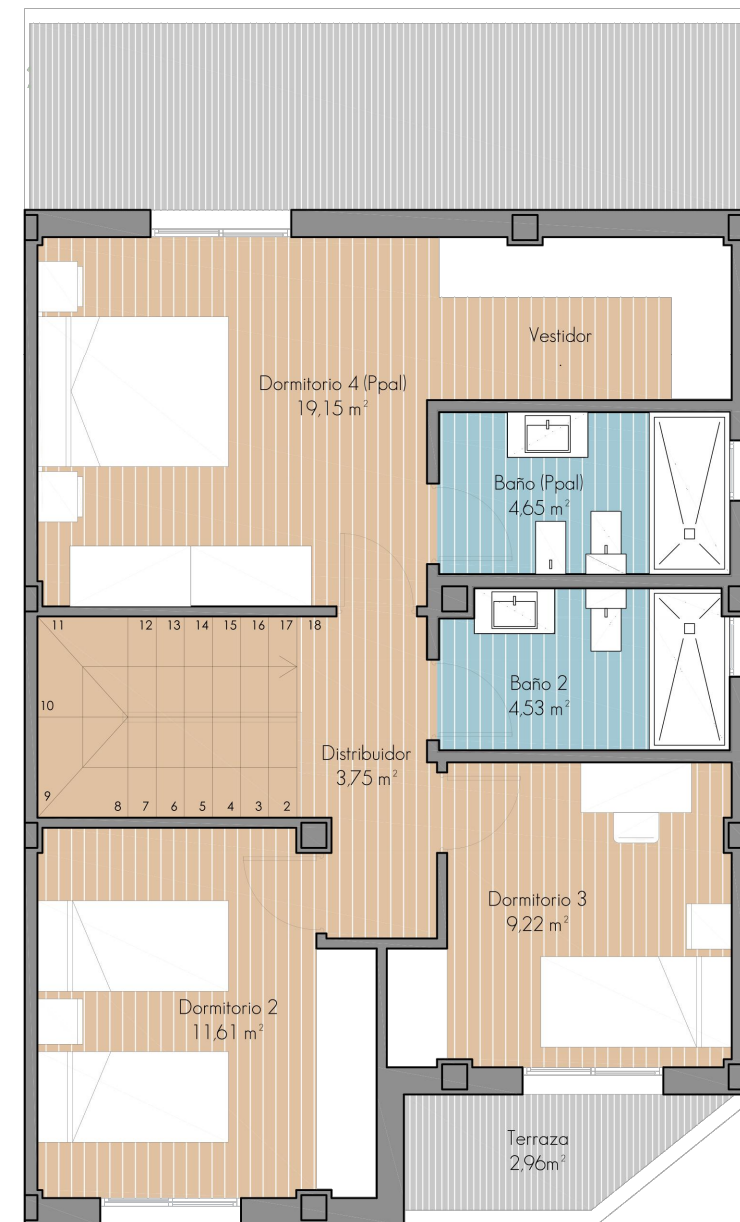
PLANTA PRIMERA - 1:75
