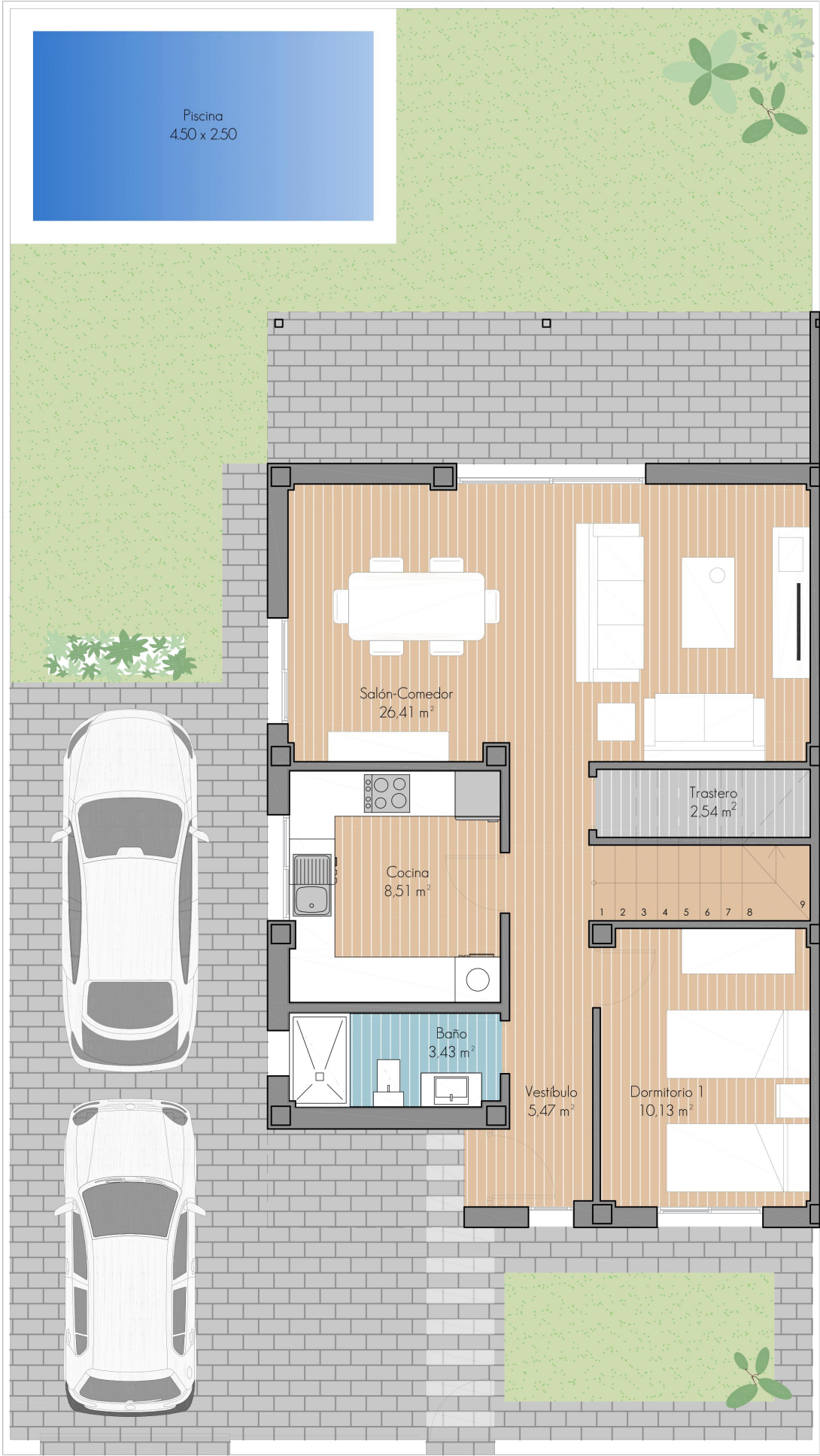
PLANTA BAJA - 1:75
