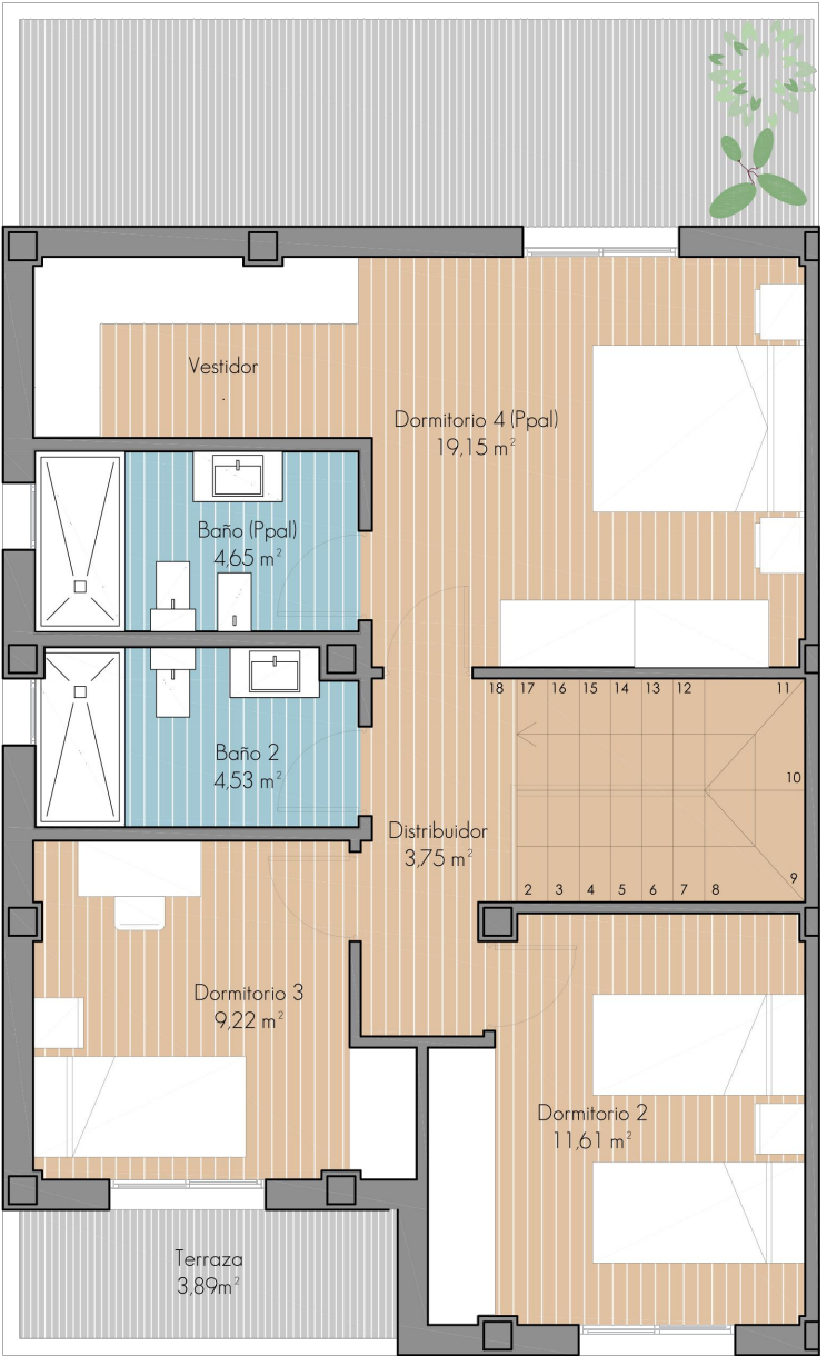
PLANTA PRIMERA - 1:75
