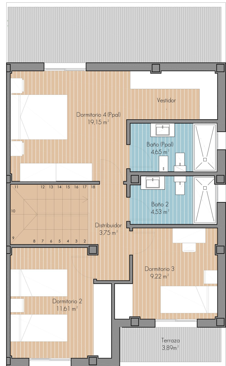
PLANTA PRIMERA - 1:75
