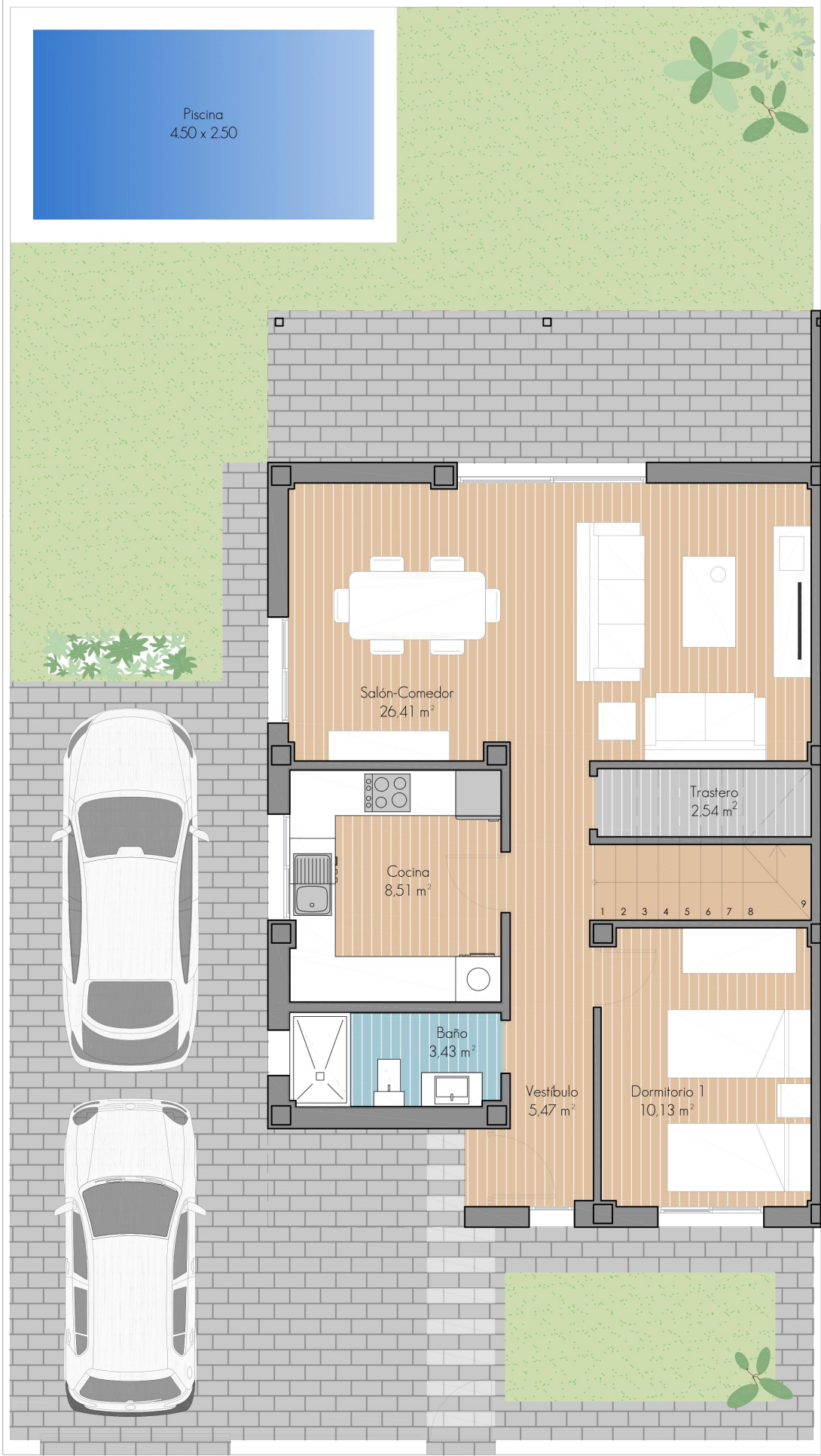
PLANTA BAJA - 1:75
