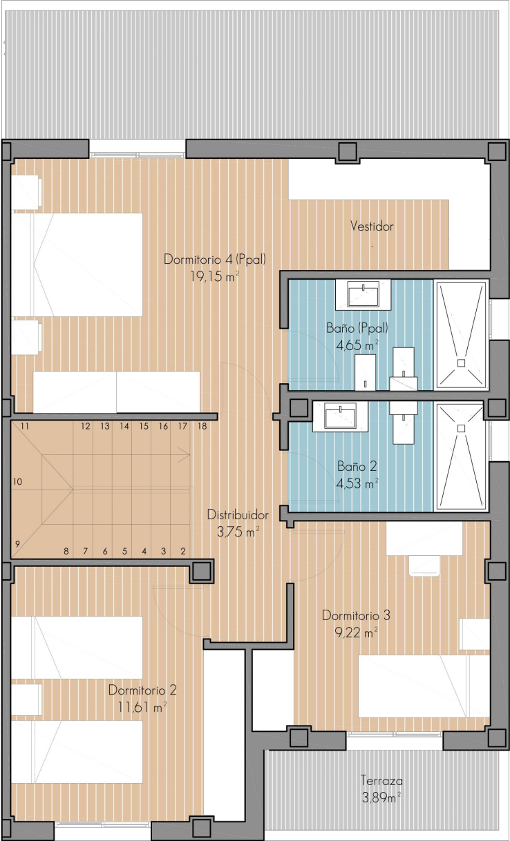
PLANTA PRIMERA - 1:75
