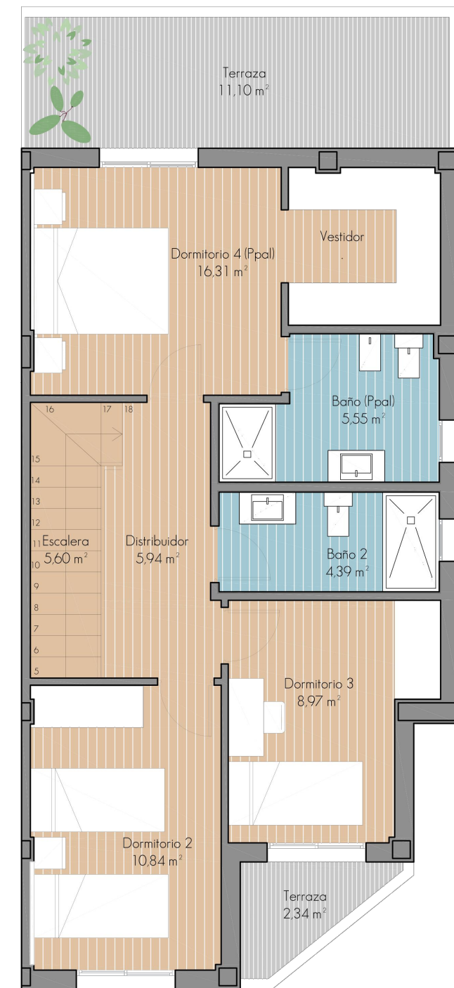
PLANTA PRIMERA - 1:75
