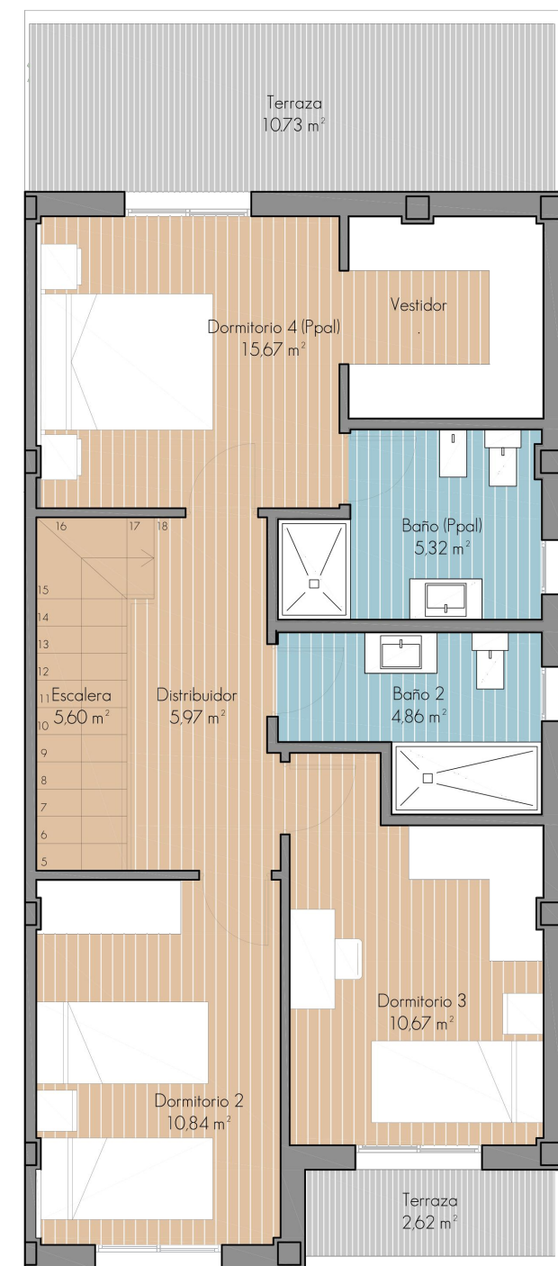
PLANTA PRIMERA - 1:75
