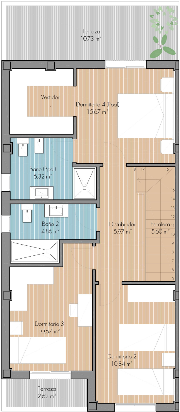
PLANTA PRIMERA - 1:75
