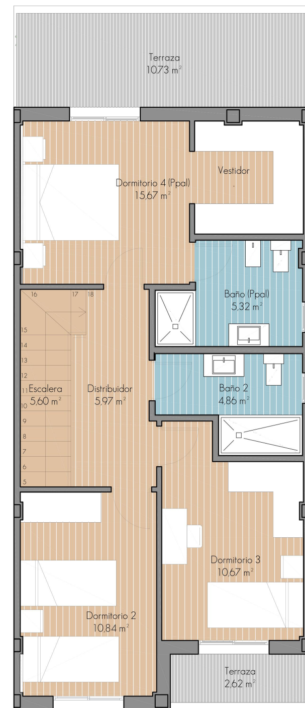
PLANTA PRIMERA - 1:75
