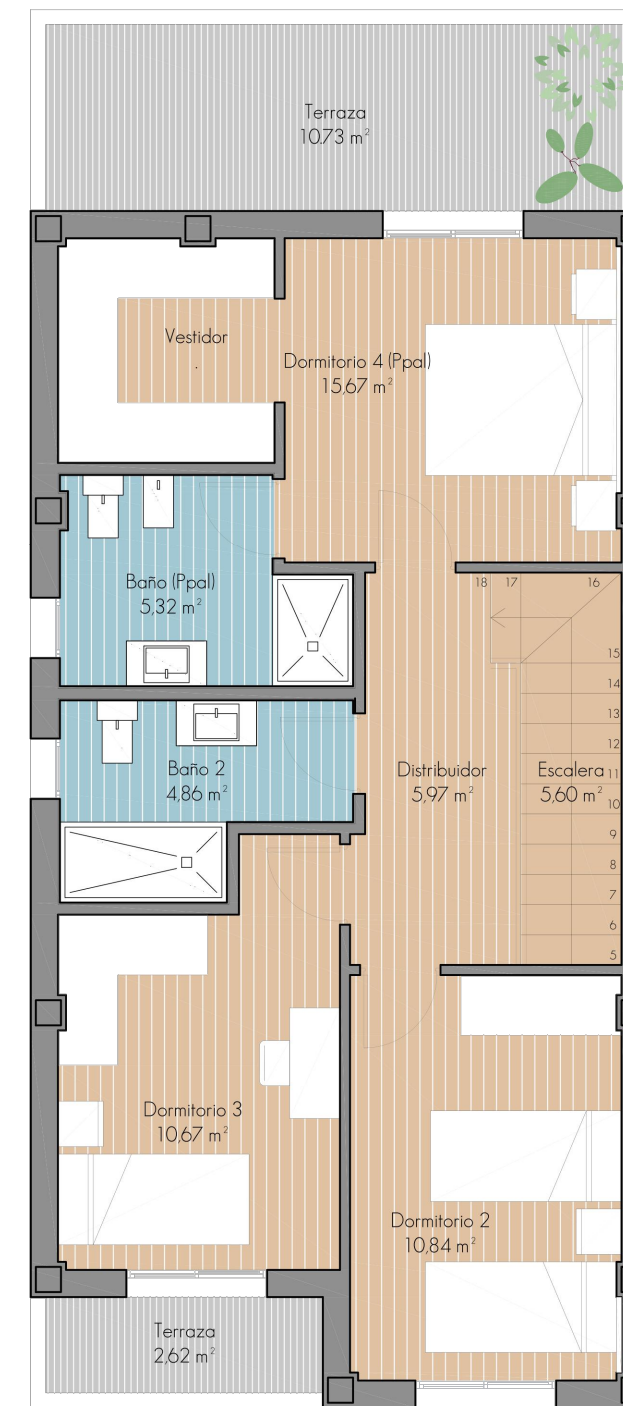
PLANTA PRIMERA - 1:75
