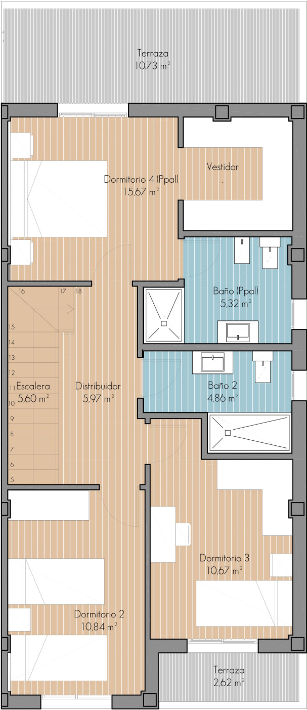
PLANTA PRIMERA - 1:75
