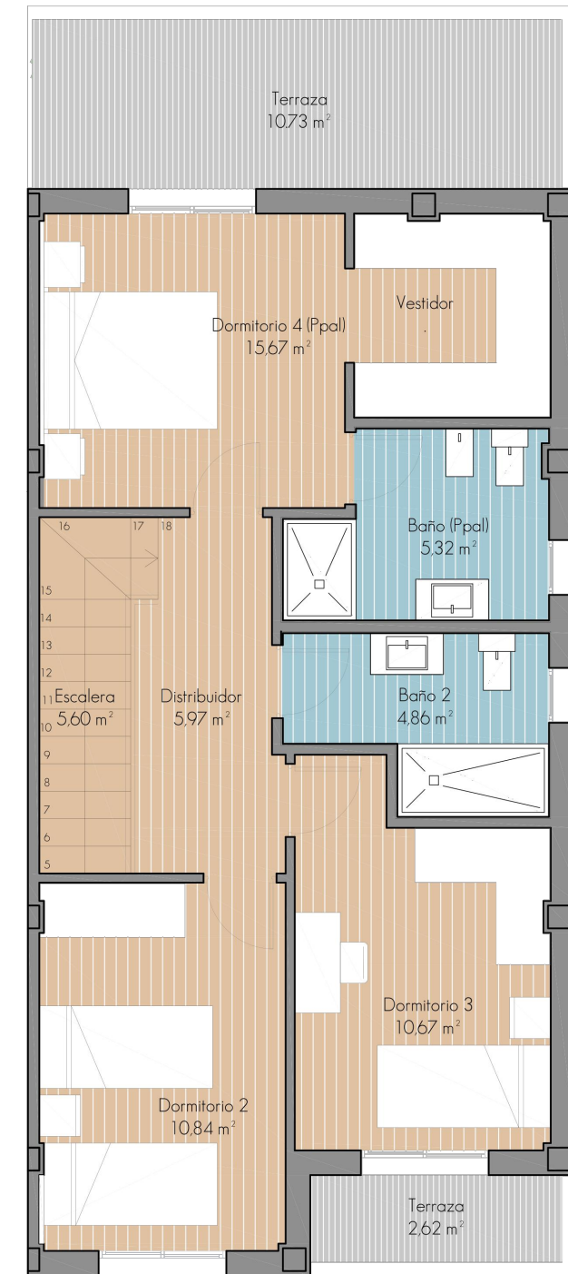
PLANTA PRIMERA - 1:75
