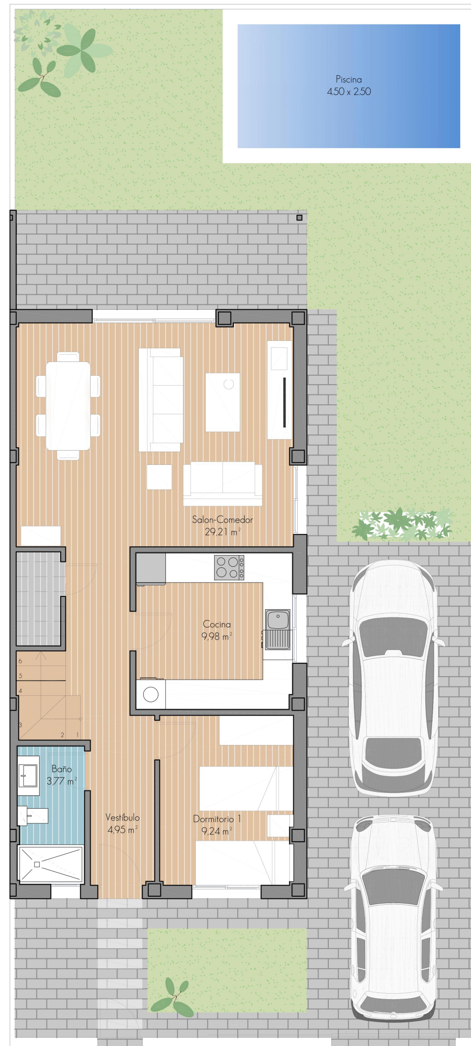
PLANTA BAJA - 1:75
