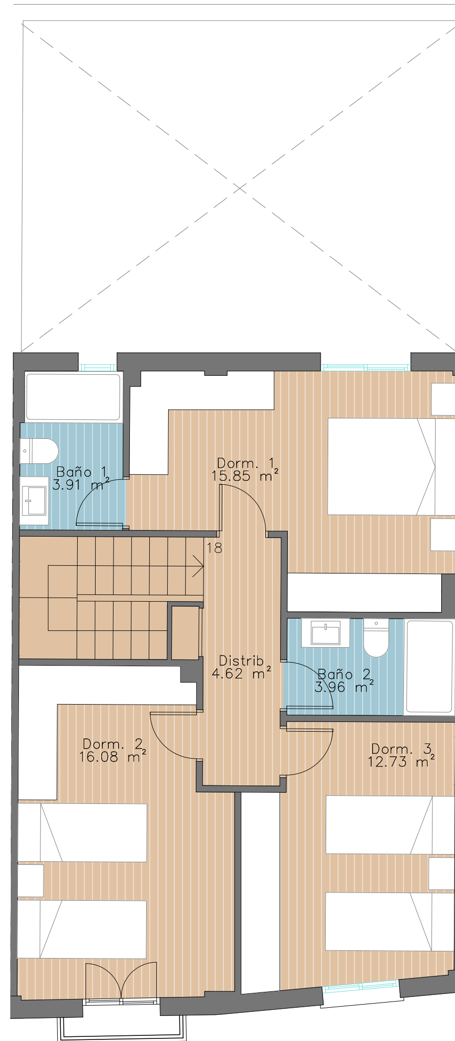
PLANTA PRIMERA
