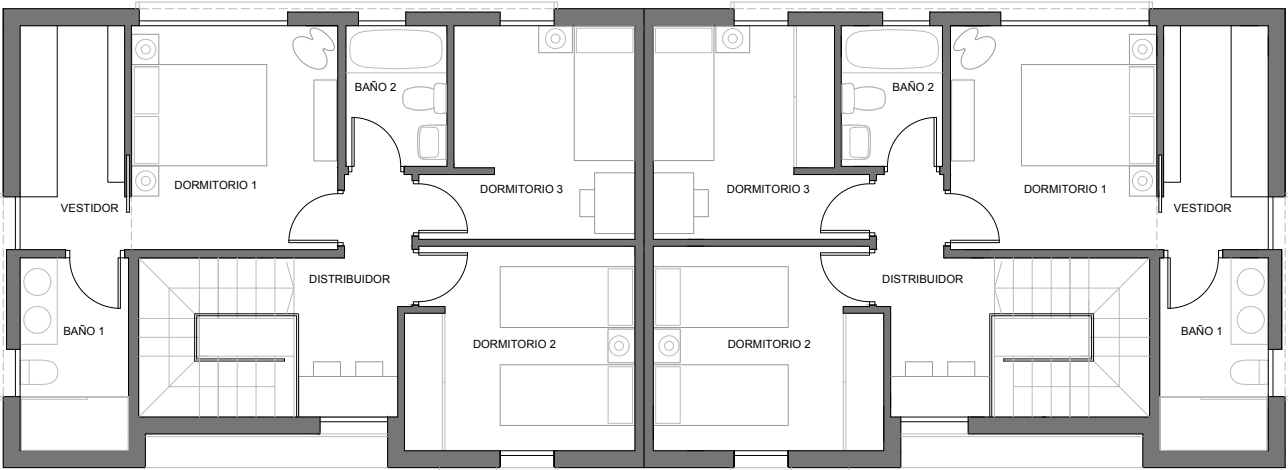
PLANTA PRIMERA
