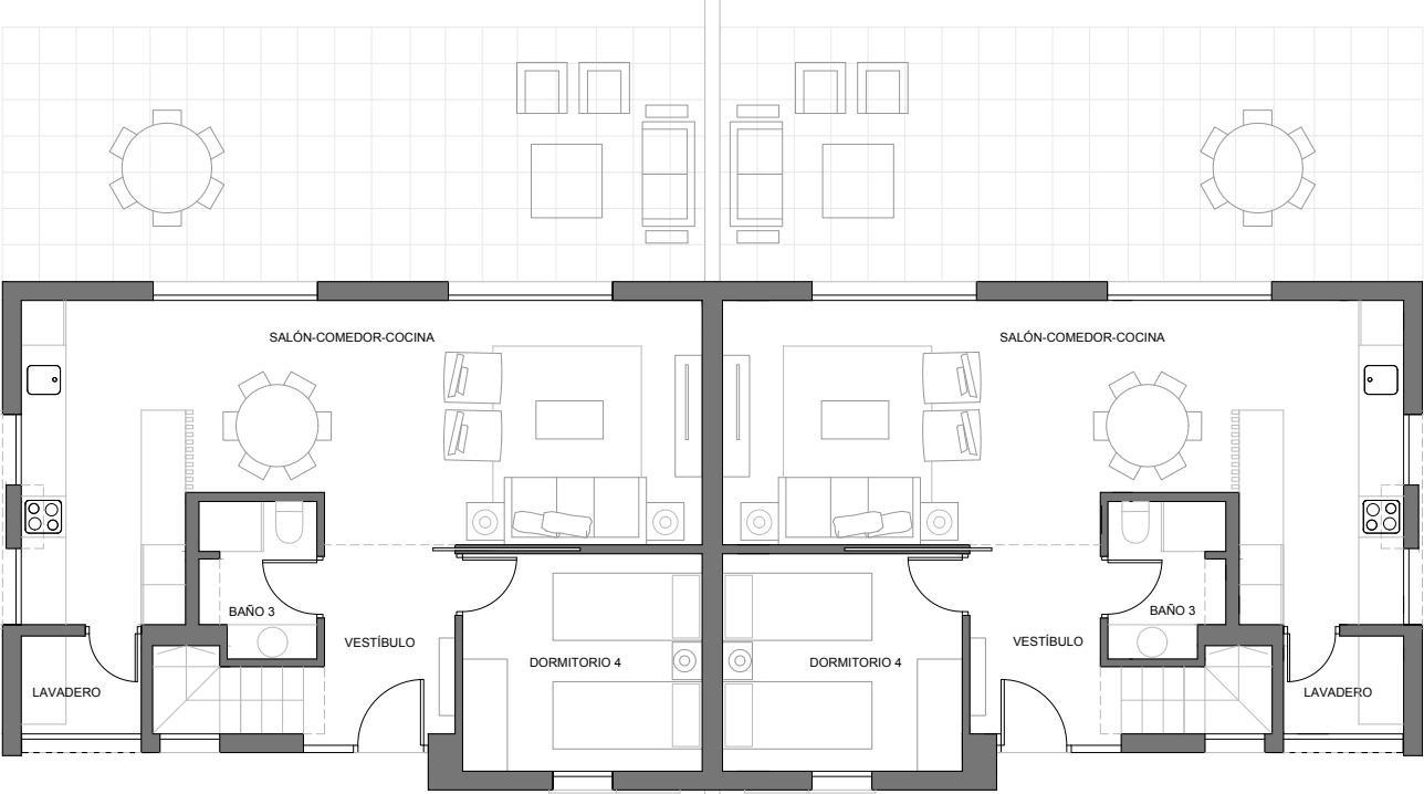
PLANTA BAJA
